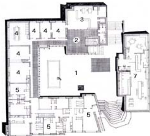
二階平面圖
