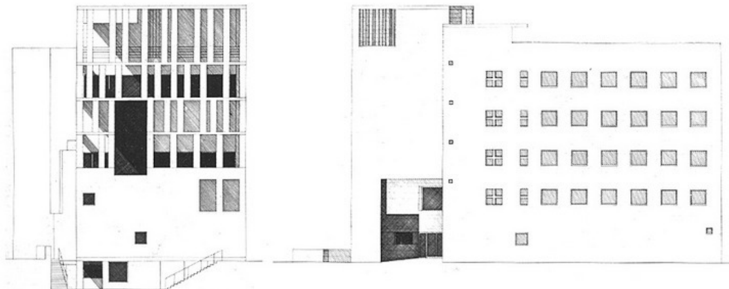
Pohledy
