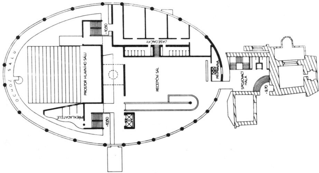
Půdorysné schéma
