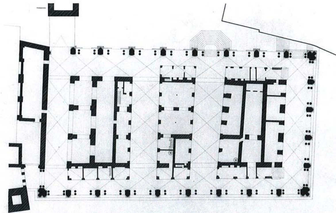
Půdorys 1 NP
