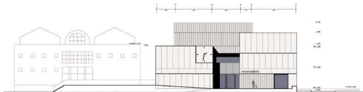
SECCIÓN POR PLAZA TRASERA.
