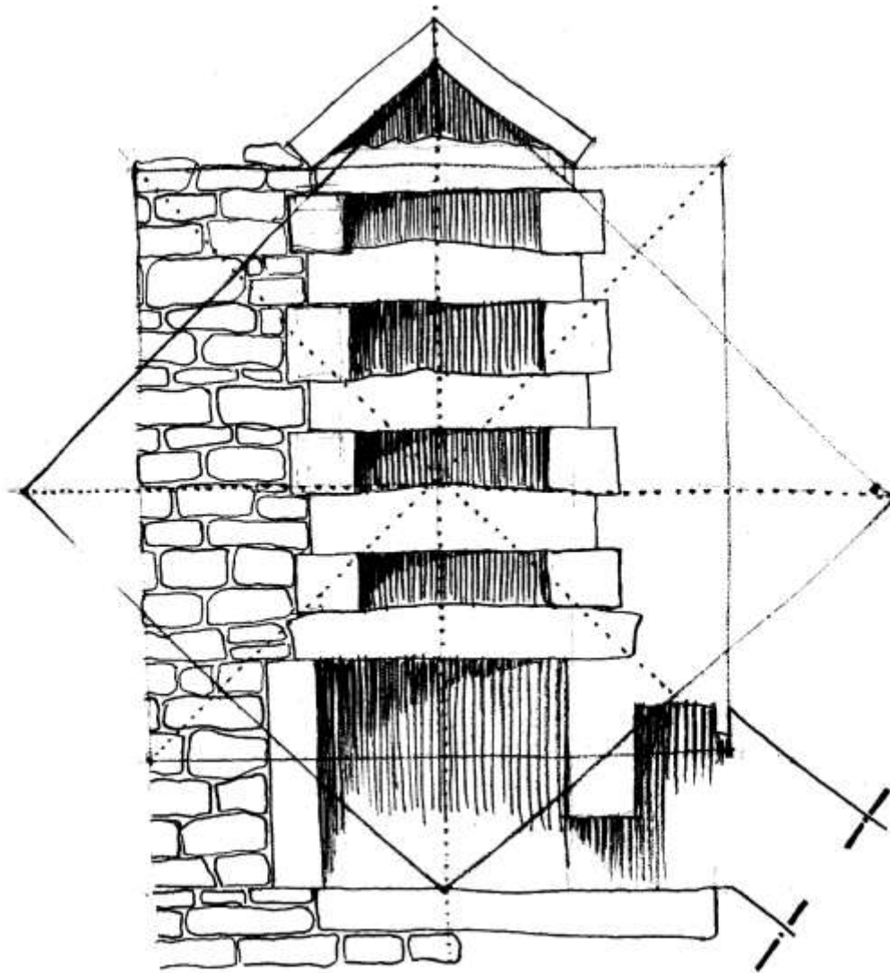
004a * řez faraónovou pohřební komorou – architrávový systém
