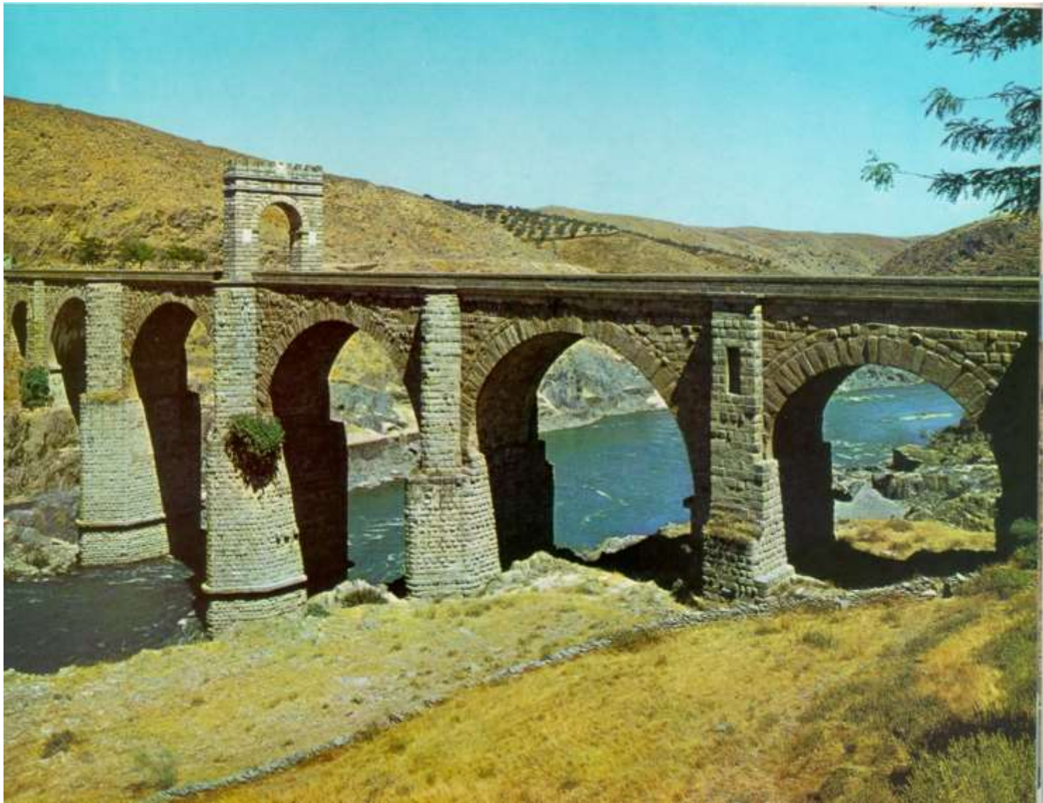
009 * Alcántarský most v Cáceres (al-quantra = arabsky most) Délka 194 m nad řekou Tajo ve výši 70 m. Vítězný oblouk na středním pilíři je zasvěcen císaři Trajánovi
