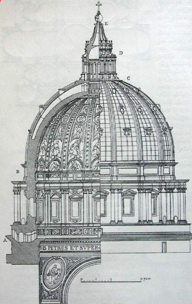
Abb. 39 Kuppel von St. Peter zu Rom (Durchschnitt und Aufriß)
