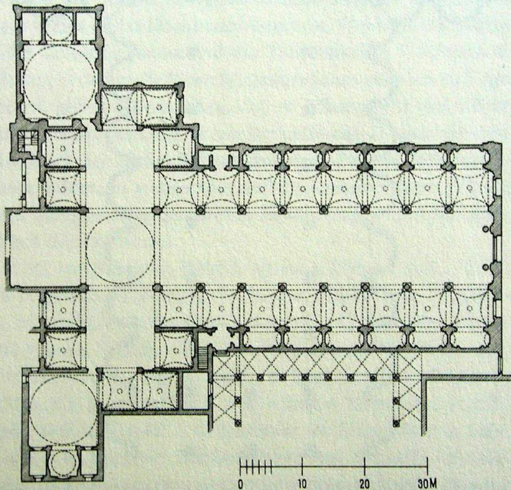
Fig. 26. Filippo Brunelleschi: S. Lorenzo, Florenz, 1418-1521
