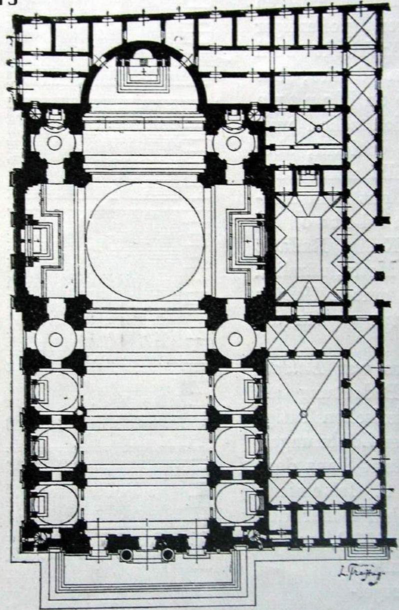
Abb. 53 Grundriß von Il Gesù zu Rom (Nach Gurlitt)
