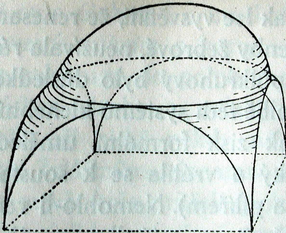
Pendantivová kopule
