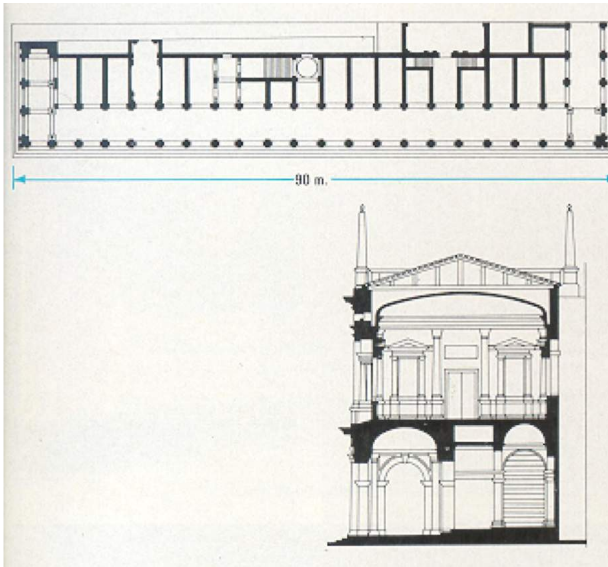
22 * Knihovna Marciany v Benátkách (1536) Jacopo Sansovino (*1486+ 1570)
